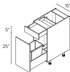
15" | BPO15
