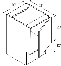
1 DOOR 18" | V18ADA
