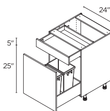
24" | BPO24
