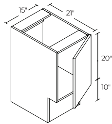
1 DOOR 15" | V15ADA
