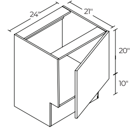
1 DOOR 24" | V24ADA
