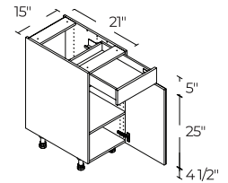
1 DOOR / 1 DRAWER 15" | V15(L/R)
