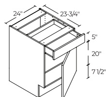
1 DOOR / 1 DRAWER 24" | B24ADA
