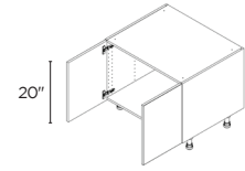
2 DOORS 30" | SBAS30 36" | SBAS36
