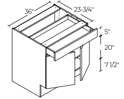
1 DOOR / 1 DRAWER 36" | B36ADA
