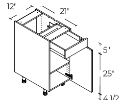
1 DOOR / 1 DRAWER 12" | V12(L/R)
