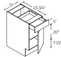
1 DOOR / 1 DRAWER 12" | B12ADA
