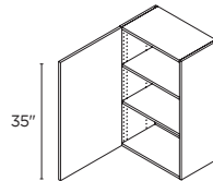
35" HIGH 1 DOOR 9" | W935(L/R) 21" | W2135(L/R) 12" | W1235(L/R) 24" | W2435(L/R) 15" | W1535(L/R) 27" | W2735(L/R) 18" | W1835(L/R) 33" | W3335(L/R)
