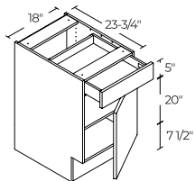
1 DOOR / 1 DRAWER 18" | B18ADA
