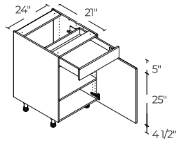
1 DOOR / 1 DRAWER 24" | V24(L/R)
