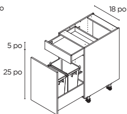
PLATEAU-TIROIR / 1 TIROIR
