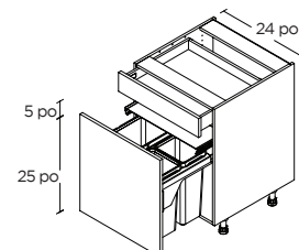
PLATEAU-TIROIR / 1 TIROIR
