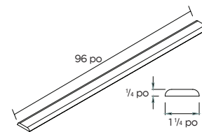
MOULURE CONTRE-PROFILÉE
